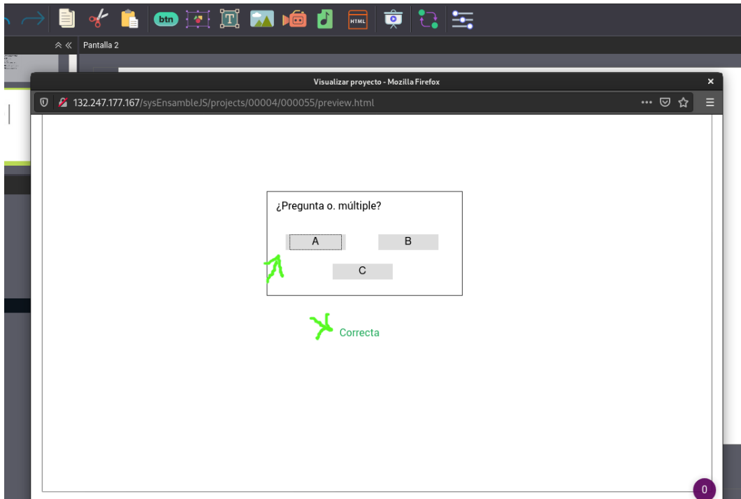
Figura 8: Al seleccionar otra opción, las realimentaciones se ocultan automáticamente.
