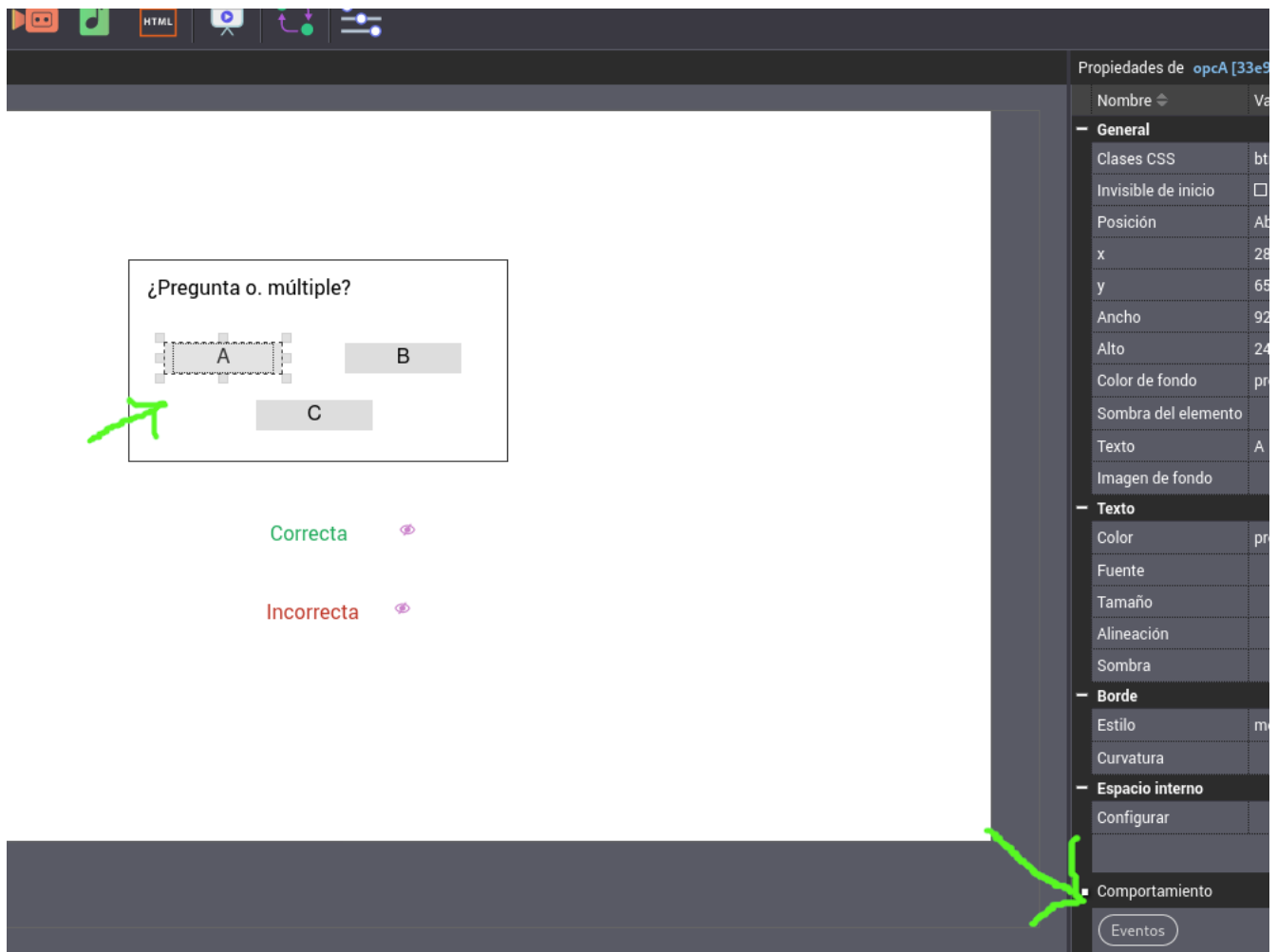
Figura 3: Seleccionamos opción y abrimos ventana de configuración de eventos y acciones.
